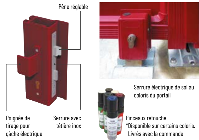
Pêne réglable
